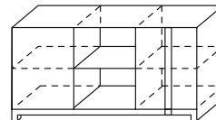
EM 202 181x42x92h
